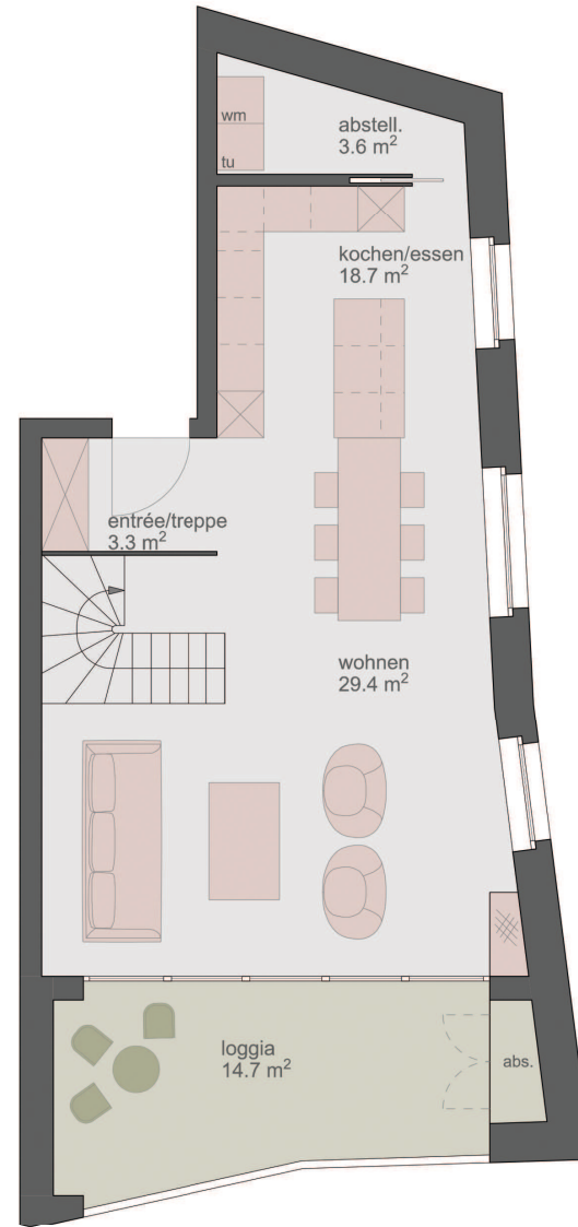
2.obergeschoss
