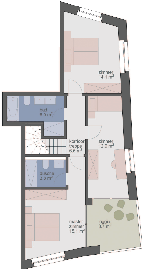
1.obergeschoss
